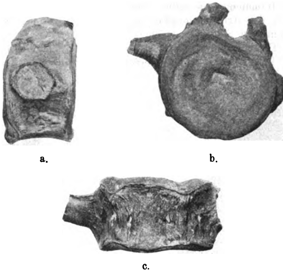
Fig. 3. Plesiosaurus Degenhardti KOKEN. \frac{2}{3} nat. Gr.
